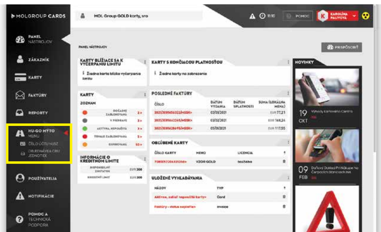
Obrázok 1: Používateľské menu
